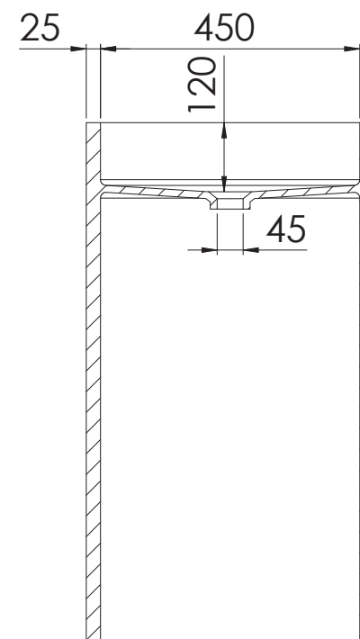
SCHNITT A-A
