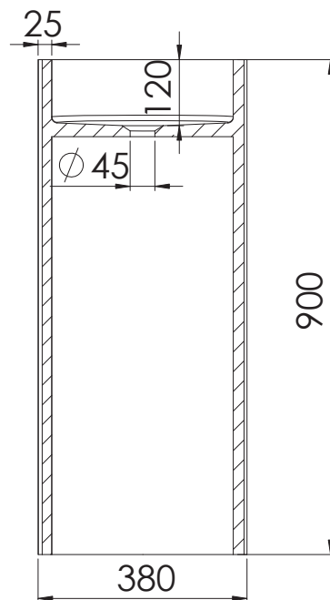
SCHNITT A-A
