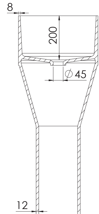
SCHNITT A-A
