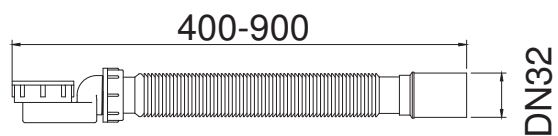
Flexibler Ablaufschlauch Flexible drain hose
