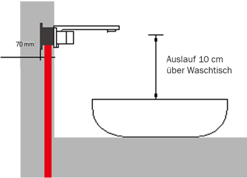
Warmwasserleitung
