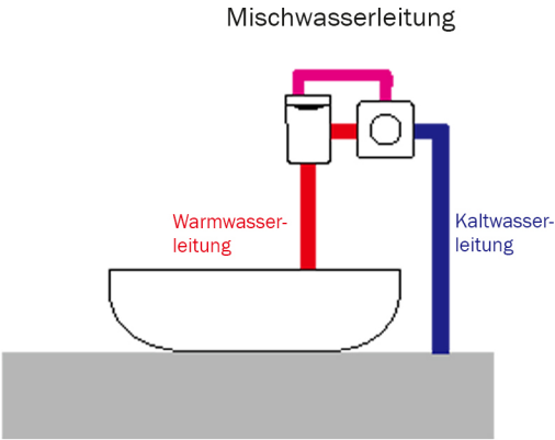
Mischwasserleitung
